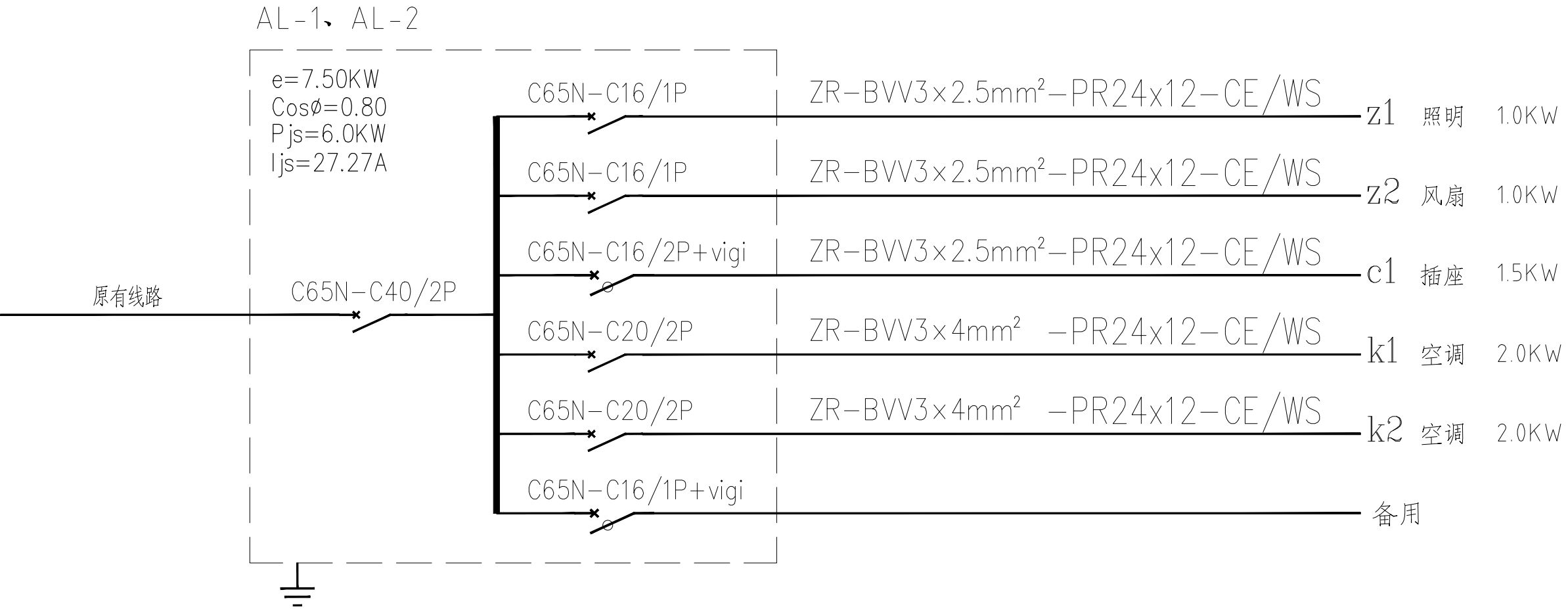
AL-1、AL-2配电系统图
